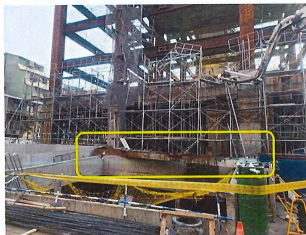
從 11 樓掉落至 1 樓之塔吊座梁 (長 100m 寬 0.3 高 0.9m)
